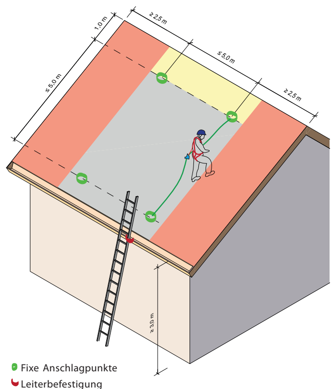
Abb. 1: Gefahrenbereiche Dachneigung < 40° (die Darstellung ist eine Empfehlung). Der erste Anschlagpunkt muss von der Leiter aus erreichbar sein. Besonderer Gefahrenbereich = rote Fläche
